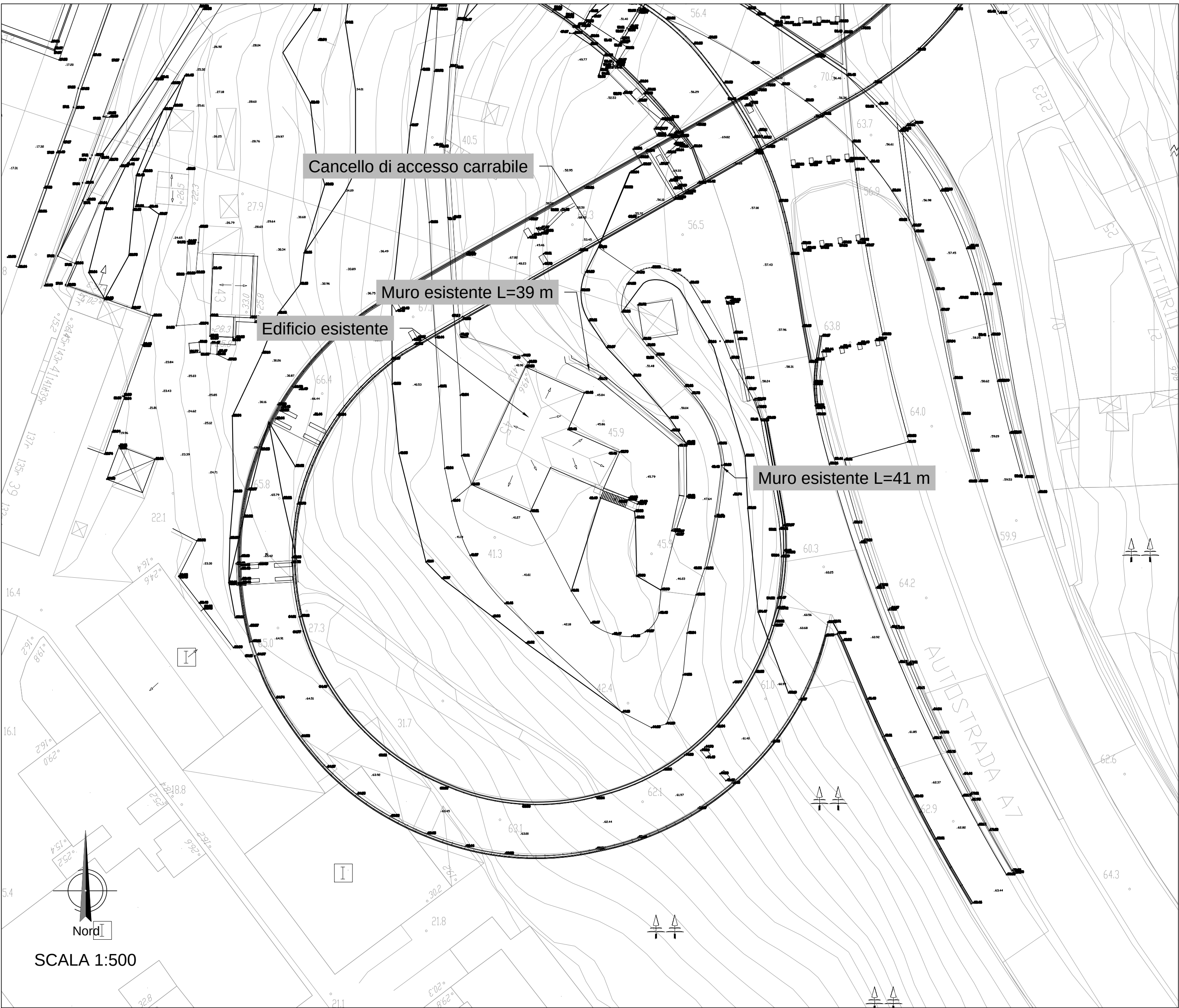
PLANIMETRIA: STATO ATTUALE
