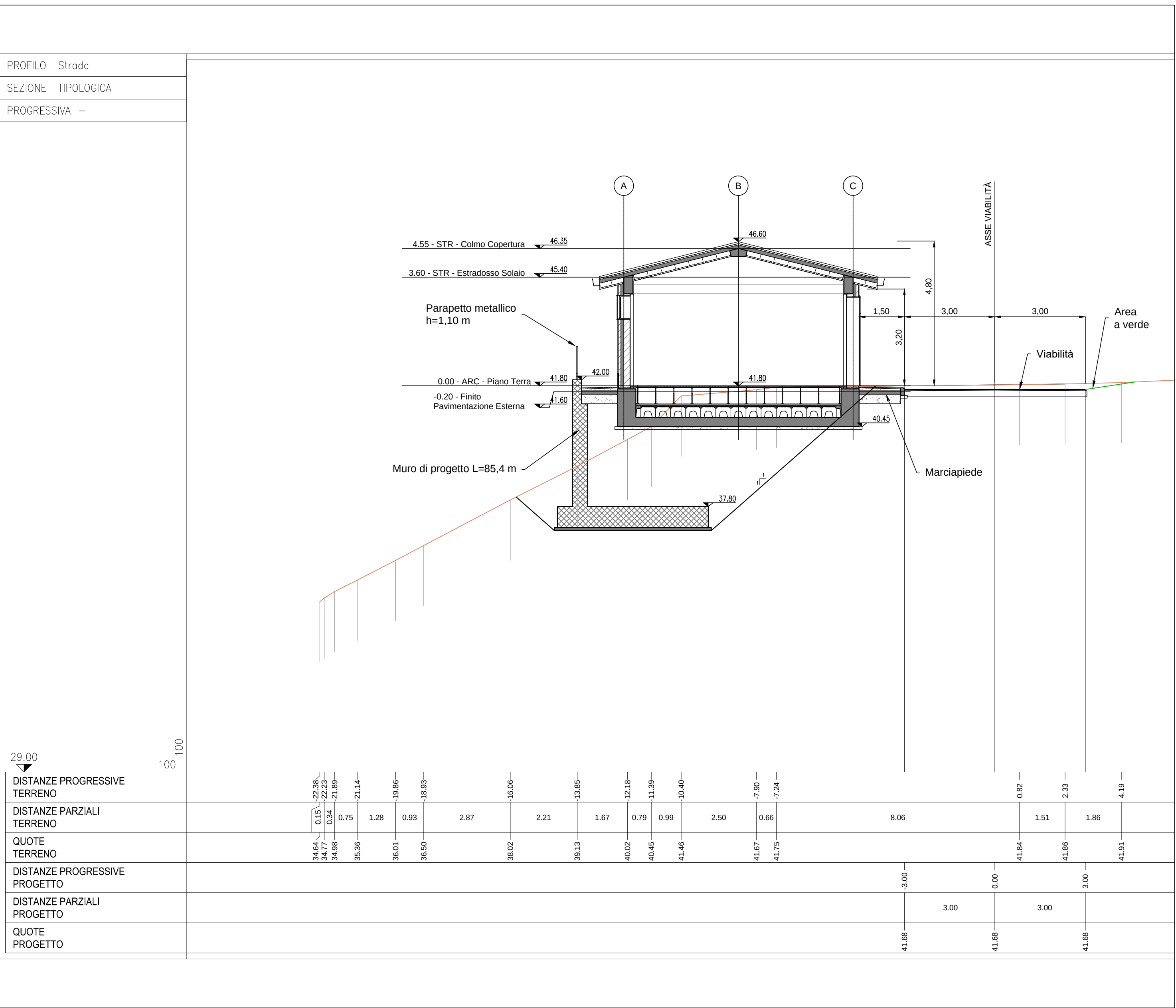
SEZIONE TRASVERSALE CARATTERISTICA (SCALA 1:100)
