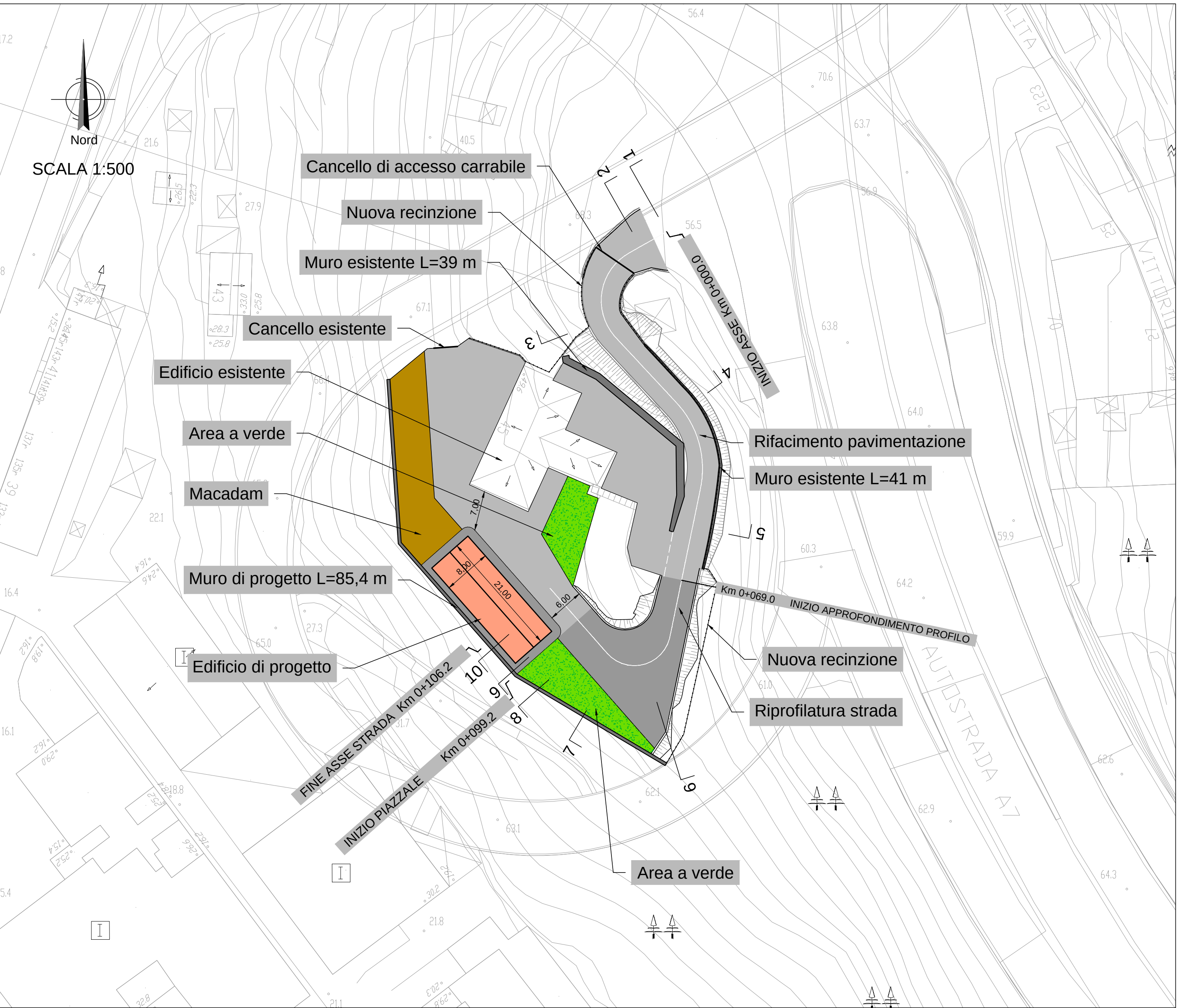
PLANIMETRIA DI PROGETTO SU BASE CARTOGRAFICA
