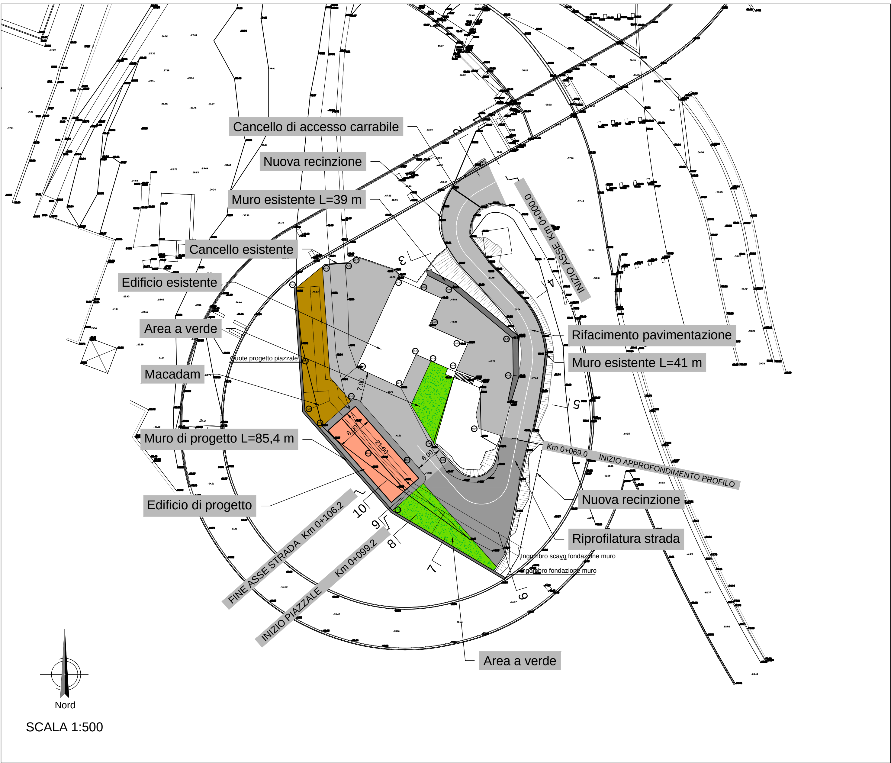
PLANIMETRIA DI PROGETTO SU RILIEVO
