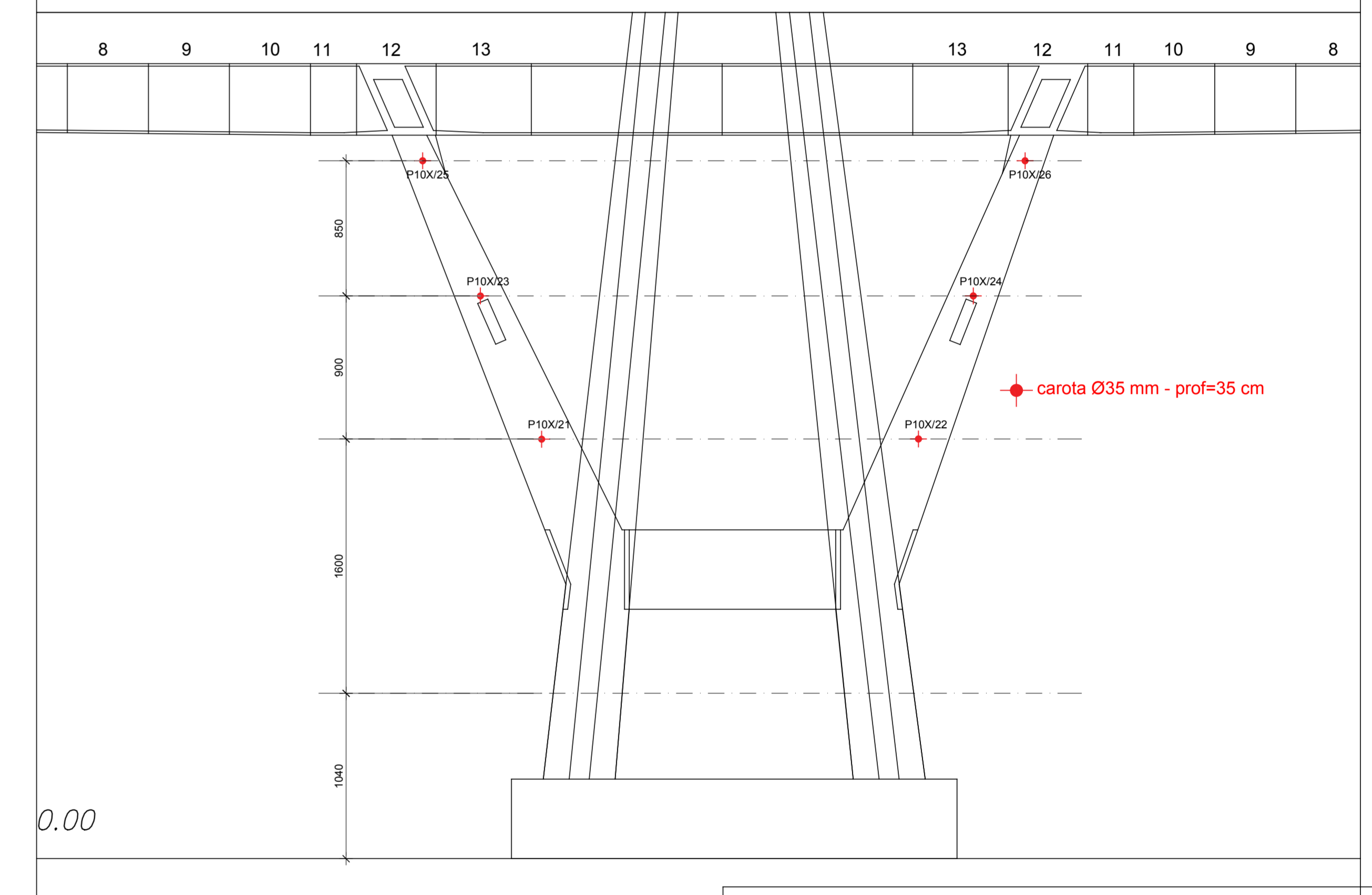
Sezione C-C
