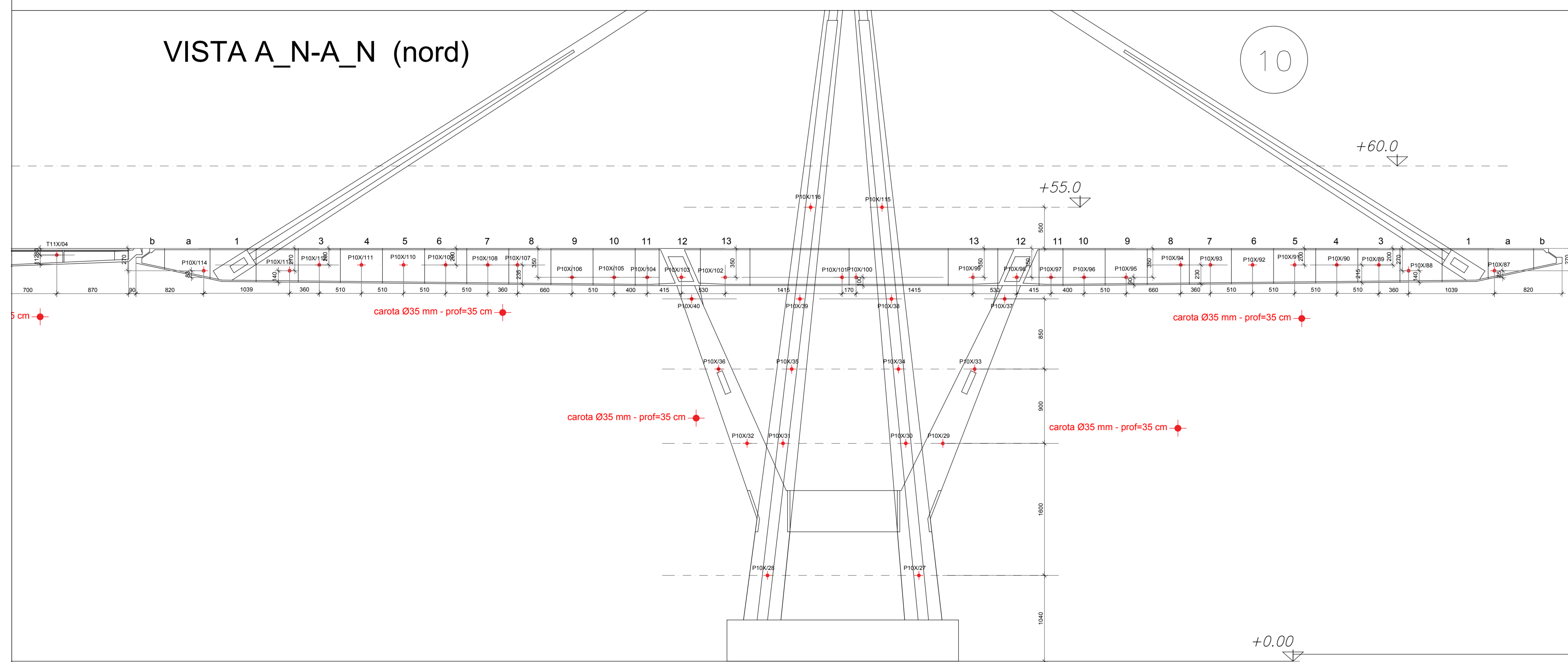
PILA 10 (impalcato)
